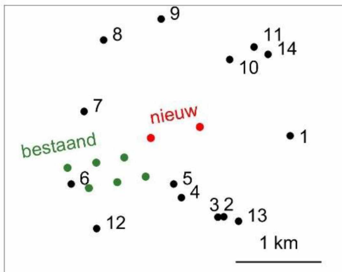
Figuur 2. Plattegrond van de zes bestaande windturbines (groen) en de twee nieuwe windturbines (rood) en de veertien toetspunten (nummers 1 t/m 14) uit het onderzoek van Pondera Consult.
