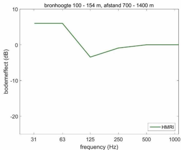
Figuur A3. Bodemeffect ( -D_{\text{bodem}} ) volgens de HMRI [18].
