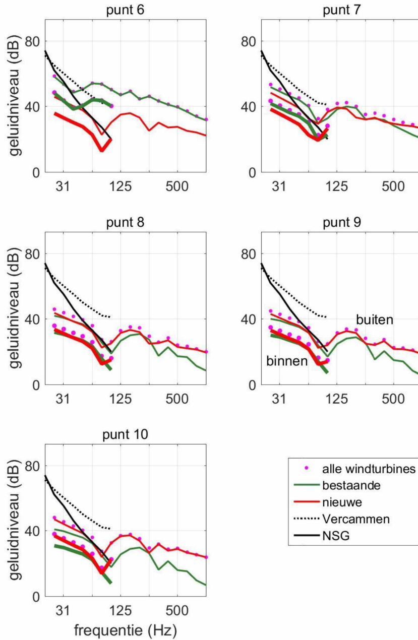
Figuur B3. Resultaten (zonder A-weging) voor de toetspunten 6 t/m 10 (dunne lijnen: geluidniveau buiten; dikke lijnen: geluidniveau binnen).
