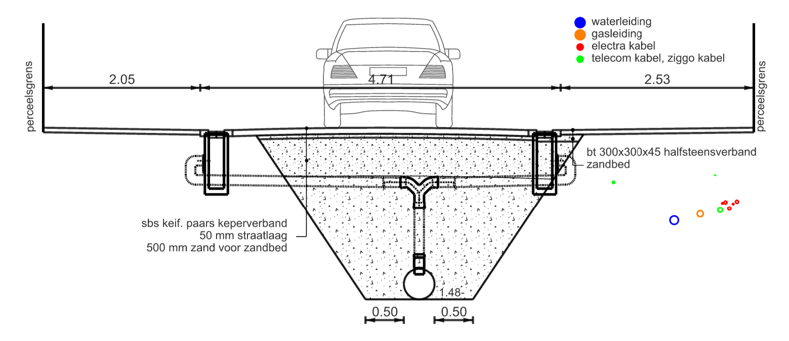
DOORSNEDE B - B' 1:50
