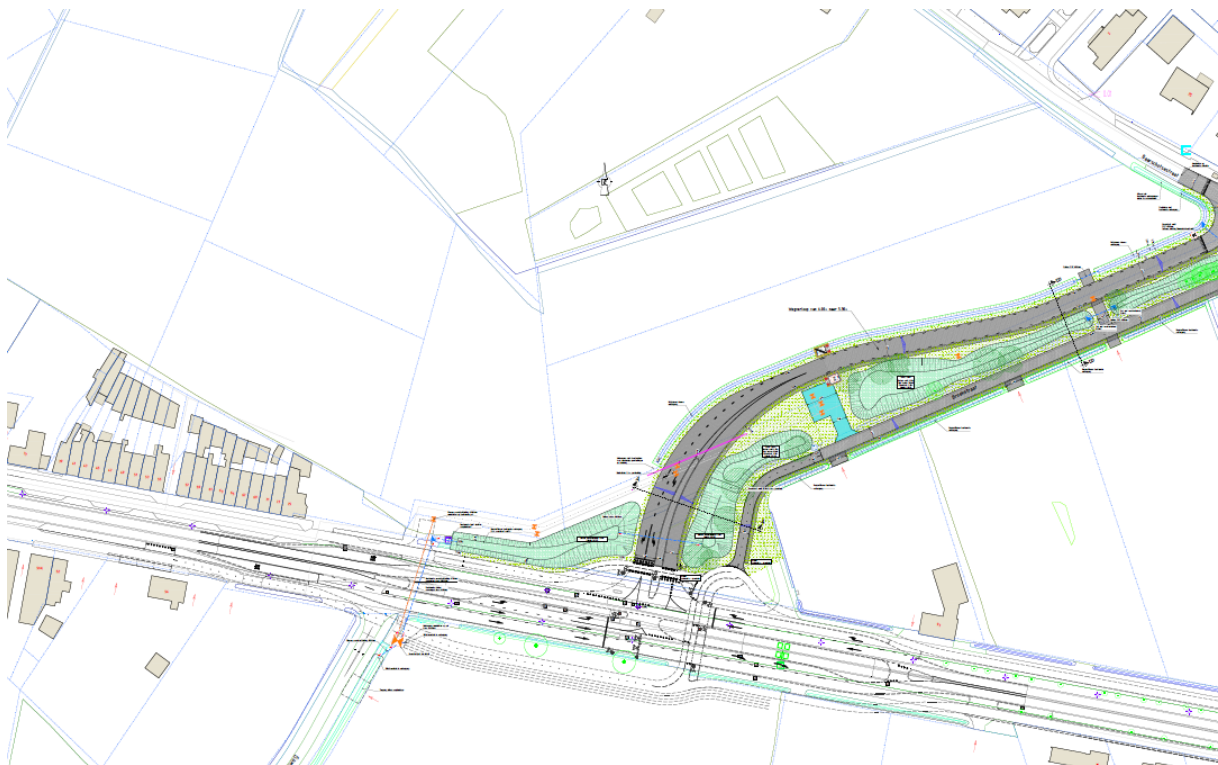
Figuur 1: Voorlopig ontwerp aansluiting Dorst-West.
